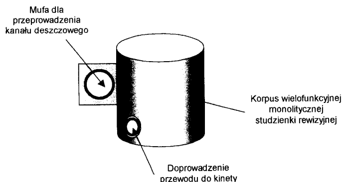
Rys. 1. Zasada funkcjonowania współczesnej kanalizacji piętrowej na przykładzie monolitycznej studzienki RSS
